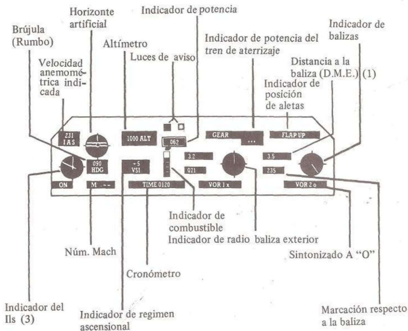
Fig. 1 Cuadro de instrumentos del puente de mando
