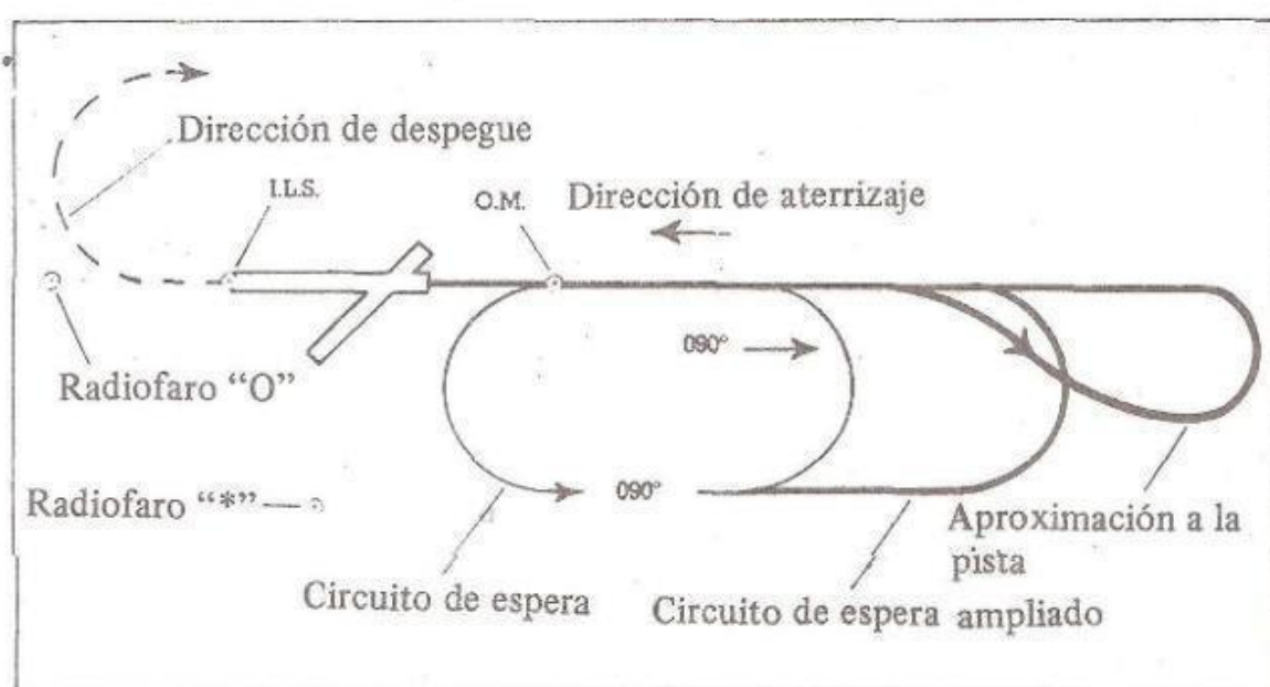
Fig. 7 Un circuito de espera característico.
